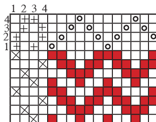
2/2 තුඩු හිරි වියමන
