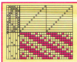
සංයෝජිත හිරි දික් නූල් වියමන් ක්‍රමය
