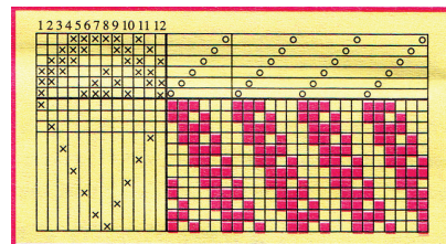
සංයෝජිත හිරි හරස් නූල් වියමන් ක්‍රමය
